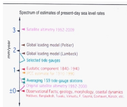
Abbildung 2 Rate der Änderungen des Meerespiegels (mm/Jahr) Das Spektrum der bis heute stattfindenden Änderungen des Meeresspiegels reicht von 0,0 mm/Jahr, jedenfalls durch beobachtete Fakten an einer ganzen Anzahl von Schlüsselorten auf der ganzen Welt, bis 3,2 mm/Jahr nach den angepassten Satellitenmessungen.
