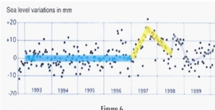
Abbildung 6 Änderungen des Meeresspiegels aus Abbildung 5 mit Berücksichtigung der ENSO-Spitze
