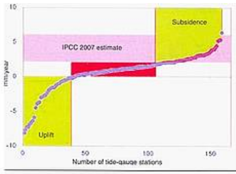
Abbildung 4 Verteilung der Raten an den 159 Messstationen der NOAA
