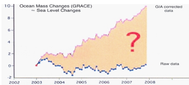
Abbildung 8 Änderungen der Wasserkonzentration aus den GRACE Satelliten Daten
