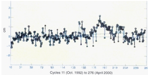
Abbildung 5 Änderungen des Meeresspiegels, beobachtet durch TOPEX/POSEIDON im Jahre 2000
