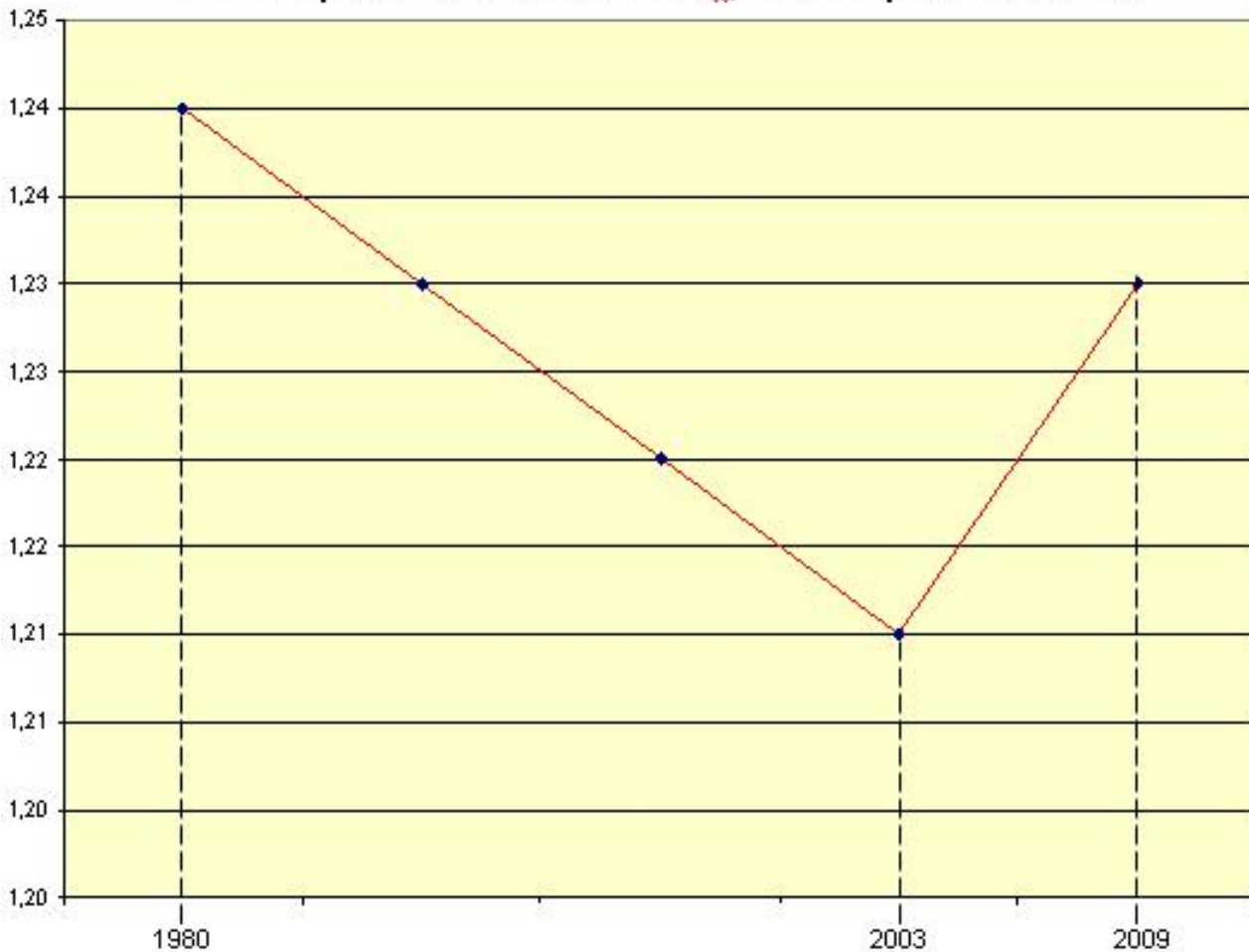
Mitteltemperatur DWD Deutschland vs Mitteltemperatur DWD HPB
