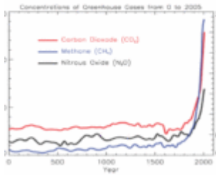
CO 2 : Entwicklung der Klimagas-Geh
