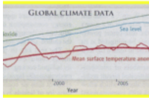
Tab: Globaler Meeres-Spiegel, nach AVISO es-Oberflächen-Temperatur, seit 2004 (ARGO) SULLO, ET. Tracking Earth's Energy, SCIENCE, Vol.328, 04.04.2010
