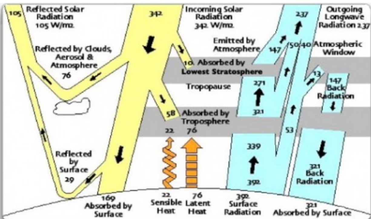
Abb. 1. Globale Energiebilanz, von Kiehl/Trenberth angepasst und erweitert. Die Werte sind Watt pro qm ( W/m^2 ). Beachte die Emission von 147 W/m^2 am oberen Atmosphärenrand (emitted by Atmosphere). Die Tropopause ist die Höhe, wo die Temperaturabnahme mit der Höhe aufhört.
