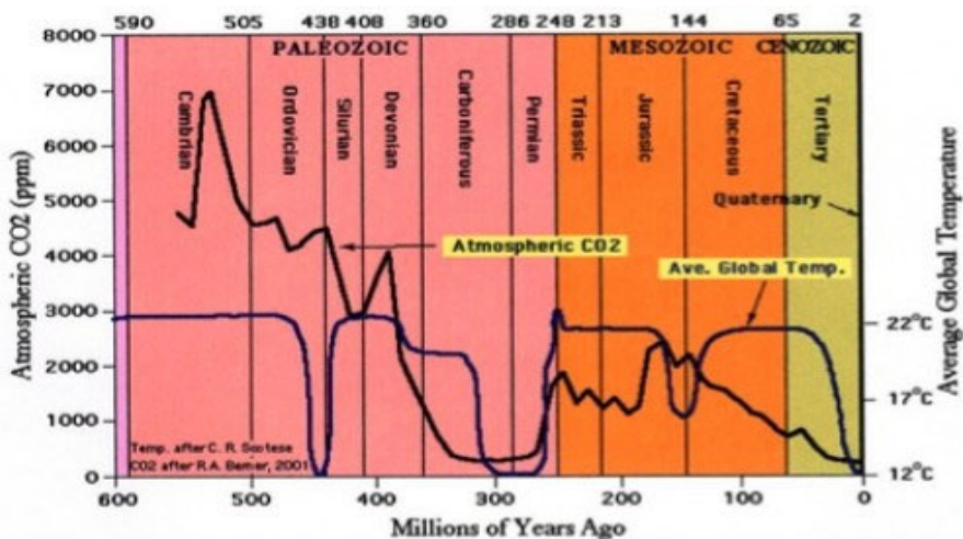
Das späte Carbon und frühe Perm (315 -270 Millionen Jahre) sind die einzigen Zeitalter in den letzten 600 Millionen Jahren mit genau so niedrigen CO 2 Werten wie heute im Quartär. Temperatur nach C.R. Scotese; CO 2 nach R.A. Berner, 2001, (Geocarb III)
