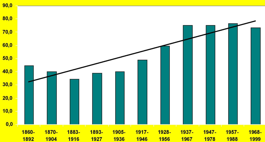
Abb.4 Mittlere Sonnenfleckenzahl über 3 Sonnenfleckenzyklen gleitend 1860 - 1999
