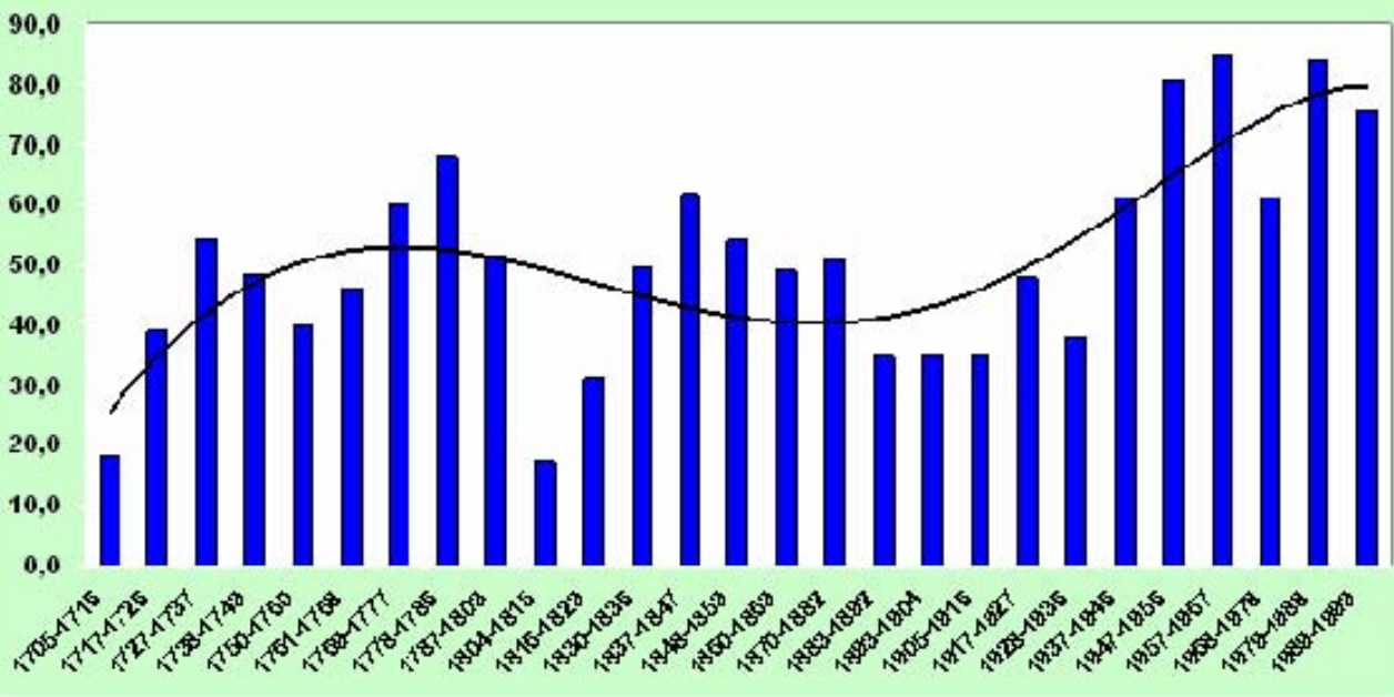
Abb. 6 Mittlere Sonnenfleckenzahl je Sonnenfleckenzyklus 1705 - 1999
