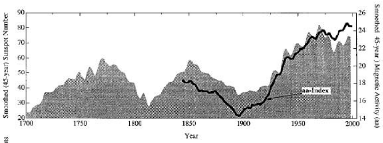
Abb. 2: 45 Jahre geglättete Kurven von Abbildung 1
