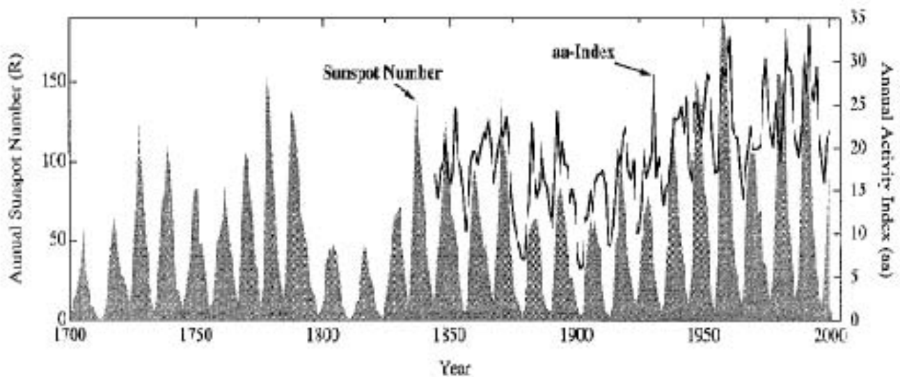
Abb. 1: Sonnenflecken und magnetische Index
